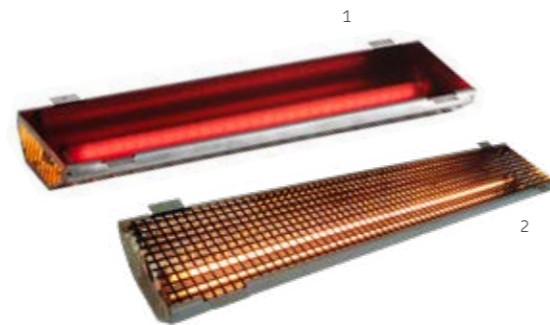
Figure 1 : radiateur ECO à vitre
