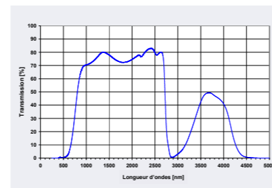
Verre sombre laissant passer le rayonnement
