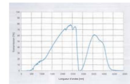
Verre blanc laissant passer le rayonnement
